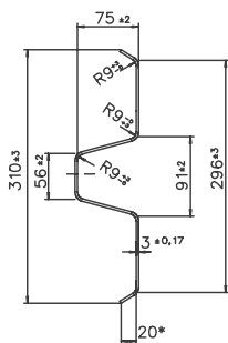
Schnitt A-A
